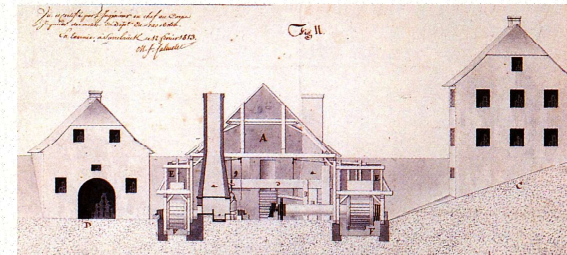
Plan de 1853 du bâtiment (A) abritant : 3 feux de forge, 2 martinets et une aiguiserie, le tout alimenté par des roues à augets
