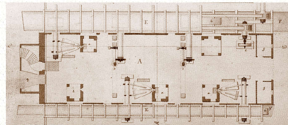
Plan de 1853 du bâtiment (A) abritant : 3 feux de forge, 2 martinets et une aiguiserie, le tout alimenté par des roues à augets
